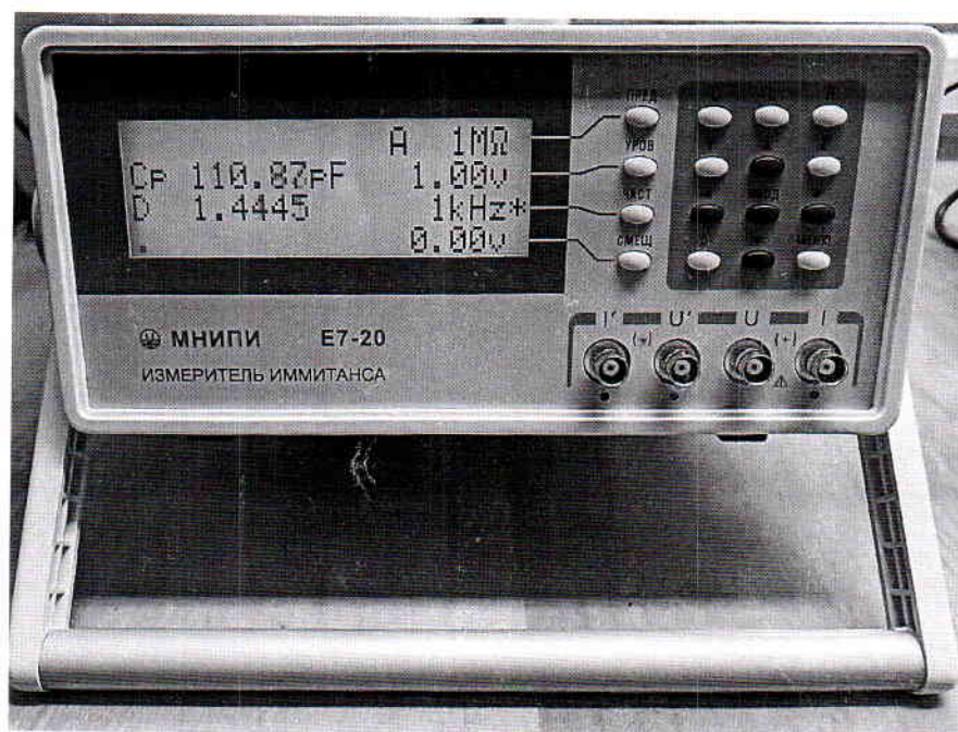
Рисунок 1.1 – Фотография общего вида измерителей иммитанса E7-20 (изображение носит иллюстративный характер)
